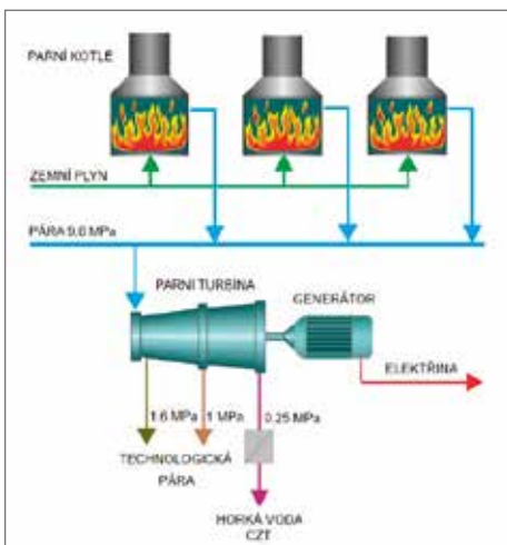
↑ Způsob výroby tepla pro vytápění a přípravu teplé vody na teplárně TAMERO INVEST s. r. o.
